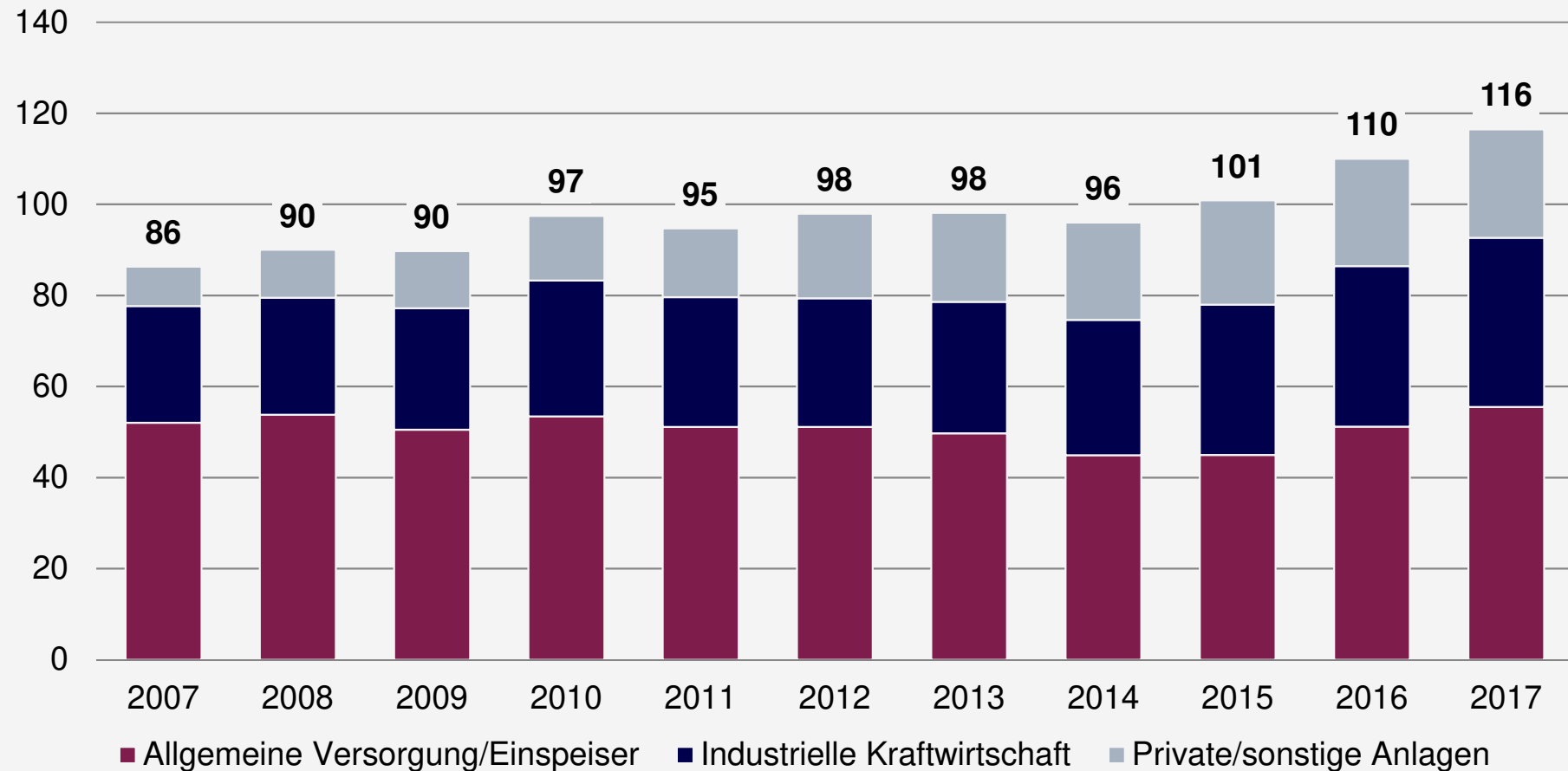
KWK-Stromerzeugung in Deutschland in Mrd. kWh
